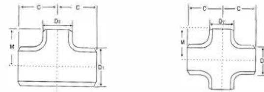
异径三通 Reducing Outlet Tee
