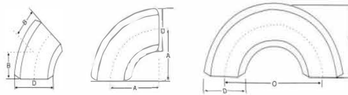
45° 弯头 45° Elbow 90° 弯头 90° Elbow 180° 弯头 180° Elbow
