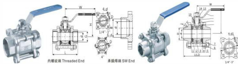
3PC不锈钢内螺纹球阀
