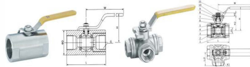
广式内螺纹球阀
