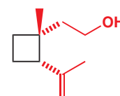
2 grandisol
