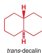
trans -decalin
