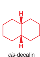
cis -decalin
