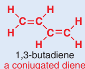
1,3-butadiene a conjugated diene
