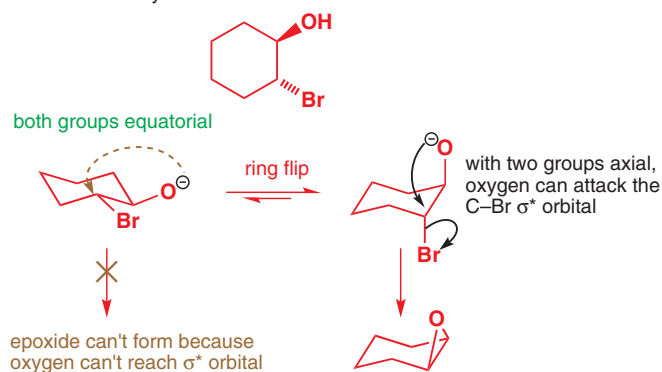
trans -2-bromocyclohexanol
