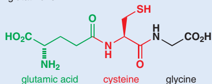
glutathione
