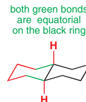
trans -decalin
