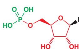
a ribonucleotide
