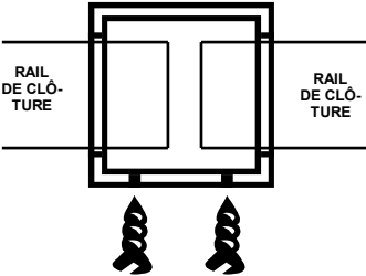
POTEAU INTERMÉDIAIRE
