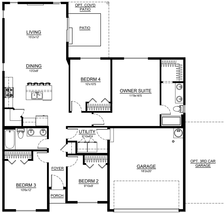
PLAN 1497
