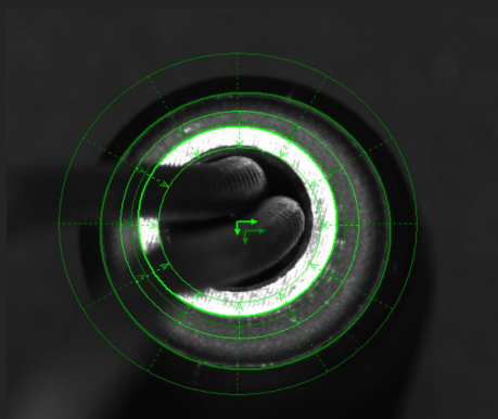
同心度測定
