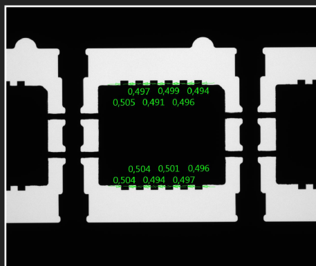
引脚距离测量
