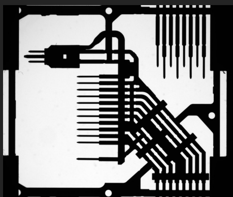
引线框架尺寸测量
