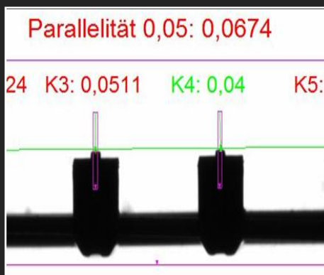
平行度測定
