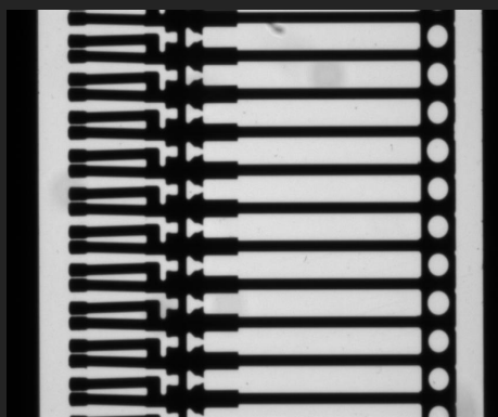
端子尺寸测量
