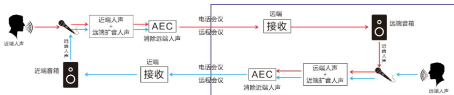
AEC原理图
