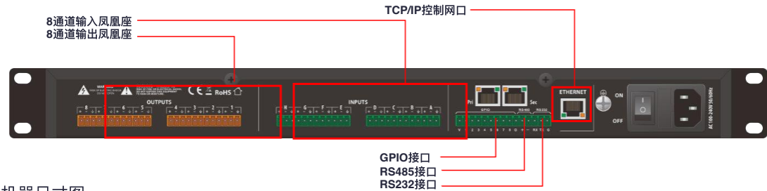
机器尺寸图
