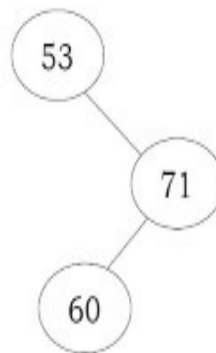
PruneBST(53,79);
