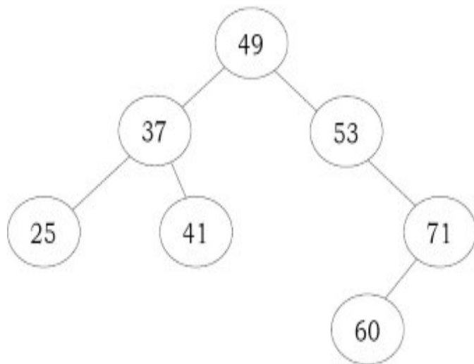
PruneBST(24,71);
