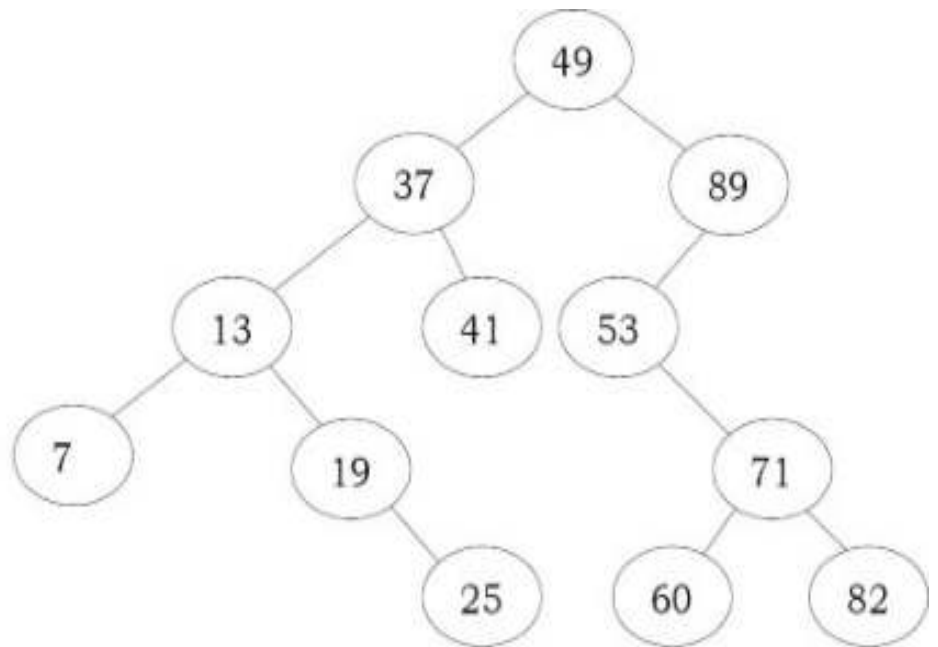
PruneBST(53,79);
