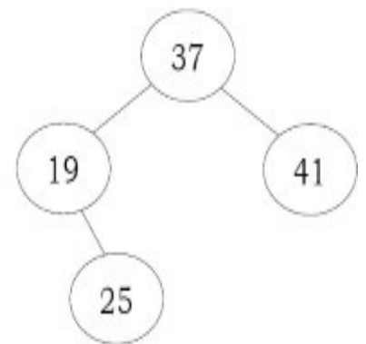
PruneBST(17,41);
