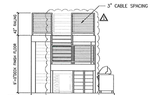
D ELEVATION SCALE: 1/4" = 1'-0"
