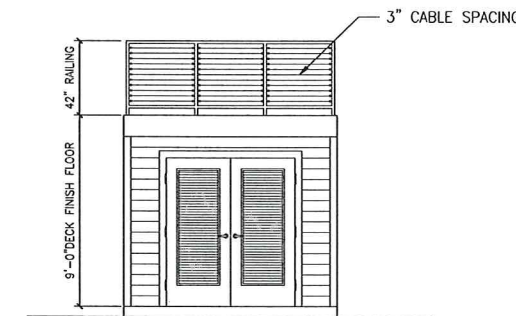
C ELEVATION SCALE: 1/4" = 1'-0"
