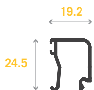
3295 Pisavidrio Curvo
