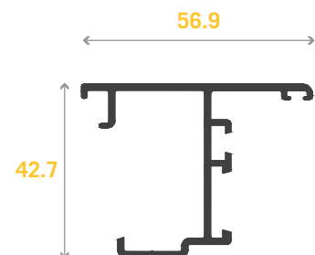
3224 Adaptador
