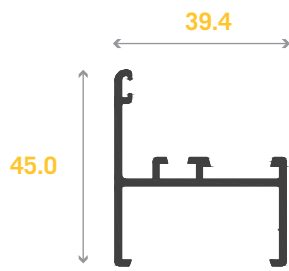
3219 Marco Perimetral
