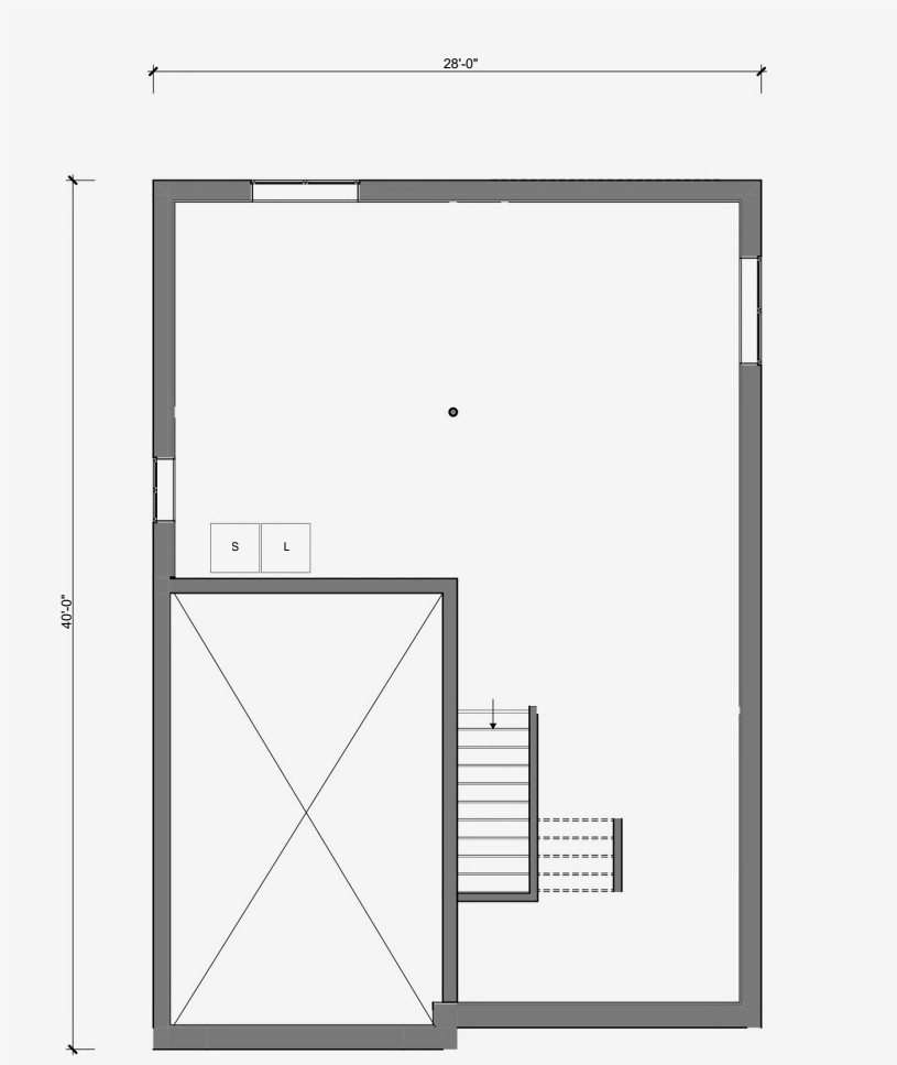
ILLUSTRATION DU SOUS-SOL
