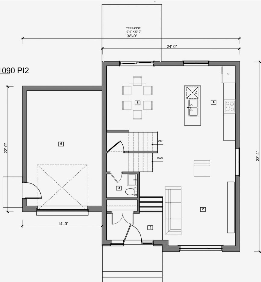
ILLUSTRATION DU REZ-DE-CHAUSSÉE
