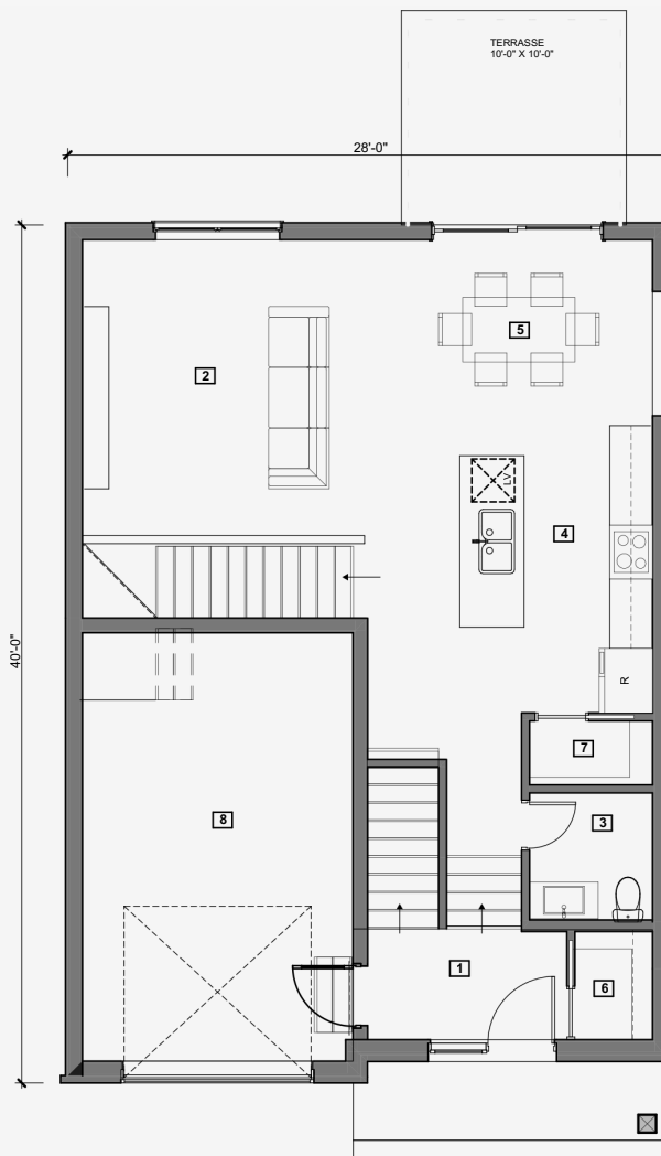
ILLUSTRATION DU REZ-DE-CHAUSSEE
