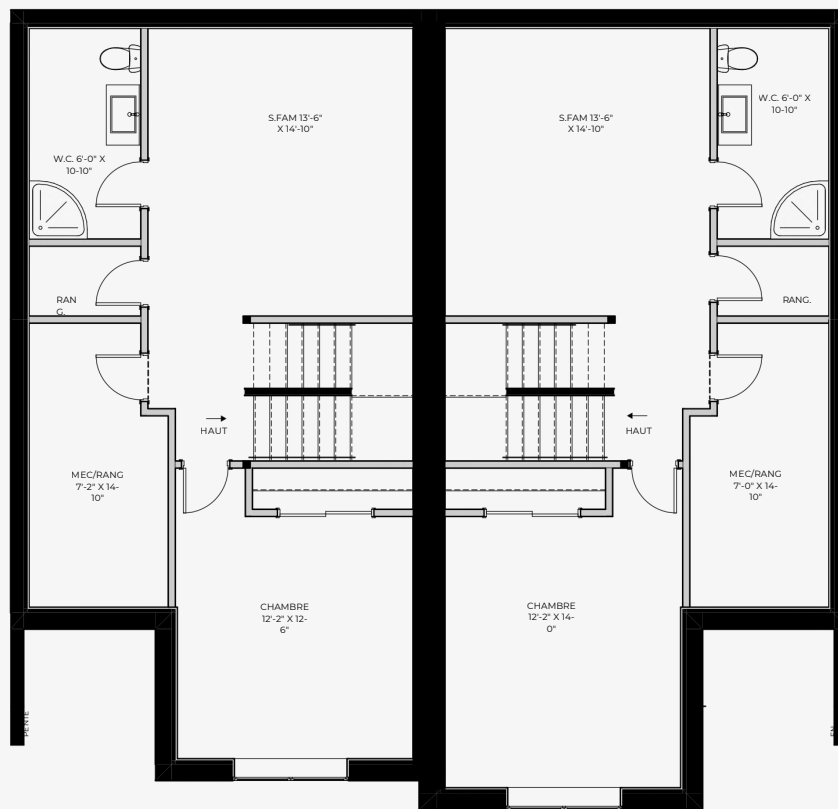
ILLUSTRATION DU SOUS-SOL
