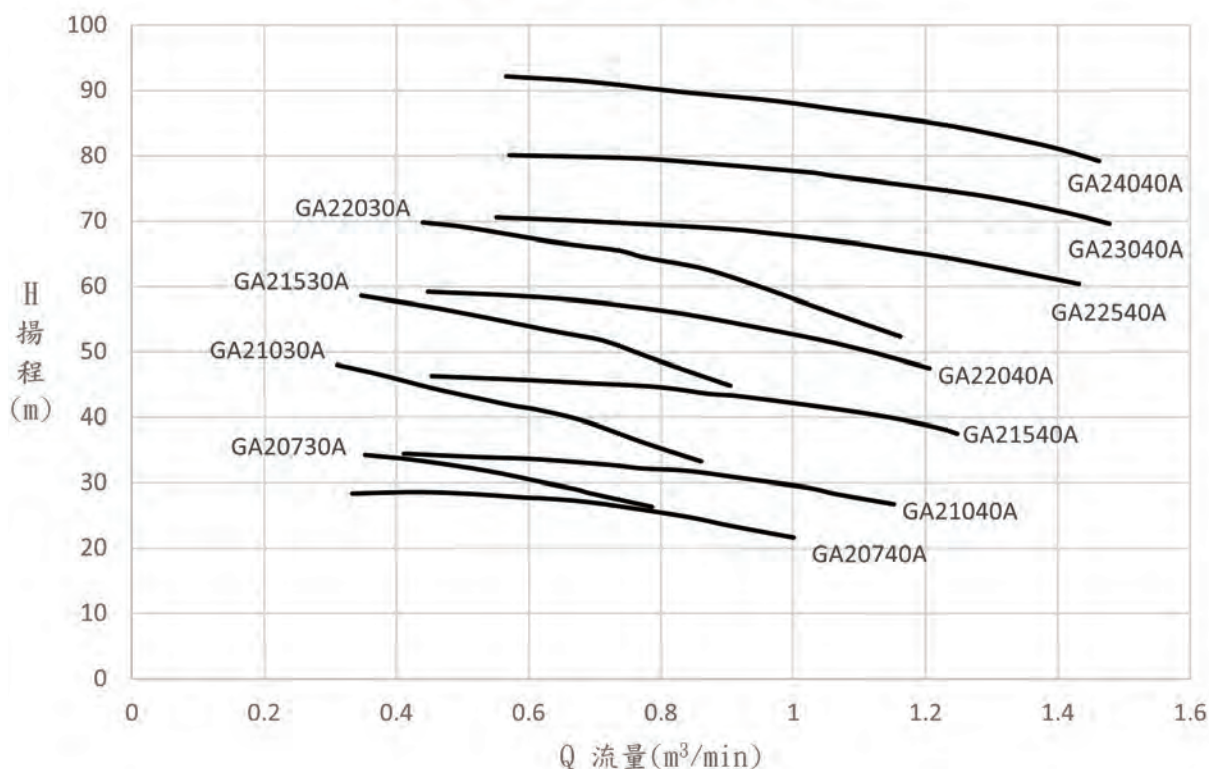
2P流量-揚程性能曲線圖(2/2)
