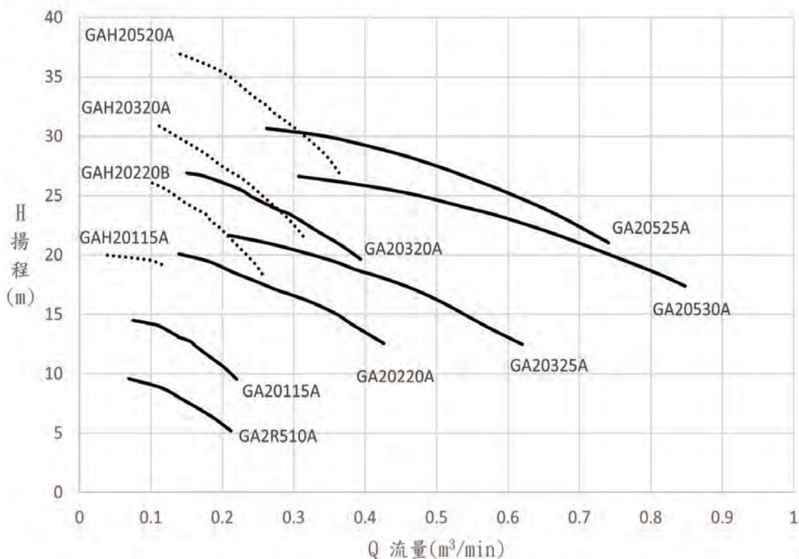
2P流量-揚程性能曲線圖(1/2)
