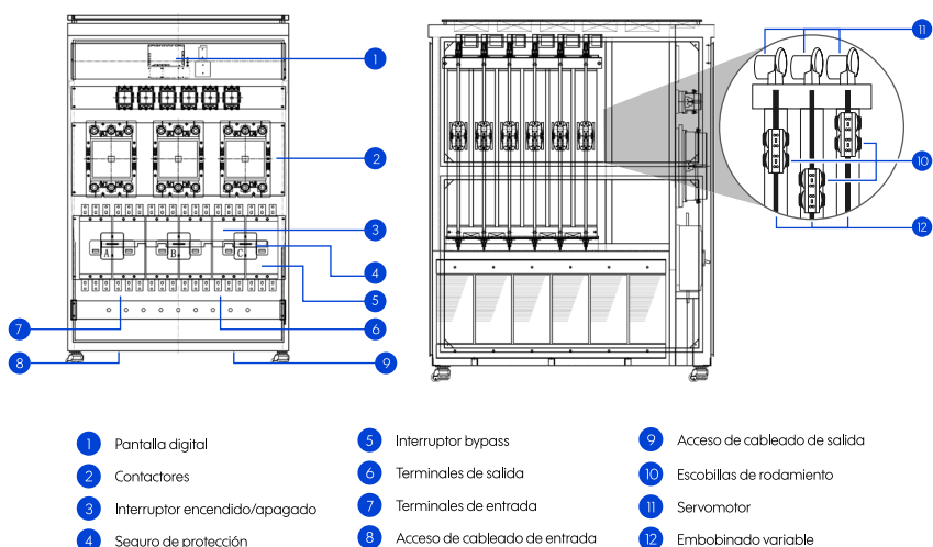
Figura 3-2 Componentes básicos AVR-IND 1300
