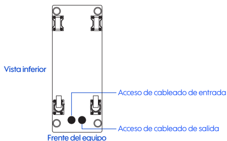
Figura 7-4 Acceso de cables de entrada y salida del AVR-IND 1300
