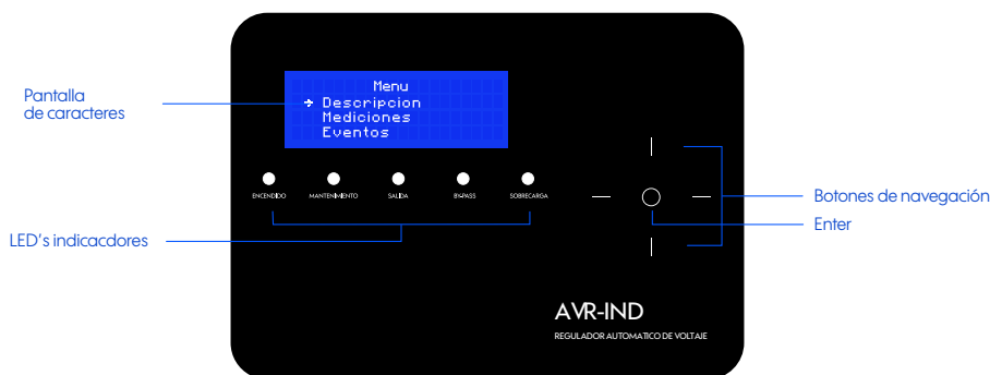
Figura 4-4 Pantalla LCD del AVR-IND 1300
