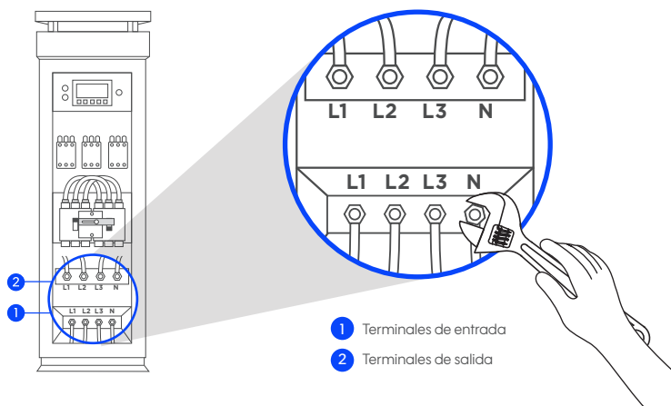
Figura 7-3 Conexiones de AVR-IND 1300
