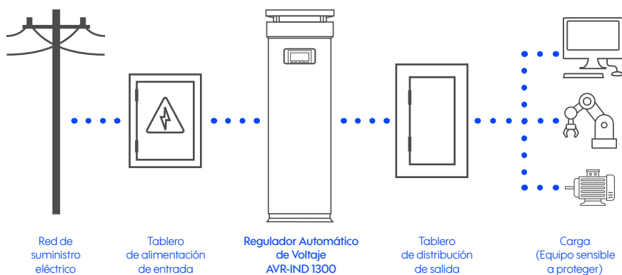
Figura 6-1 Diagrama de la instalación física del AVR-IND 1300
