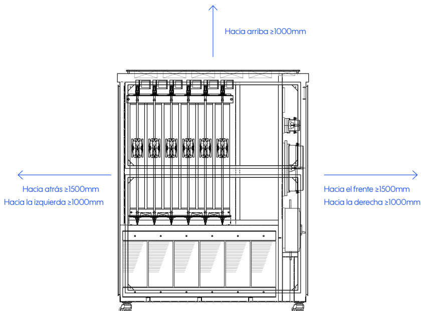
Figura 3-1 Requerimiento mínimo de espacio de instalación del AVR-IND 1300
