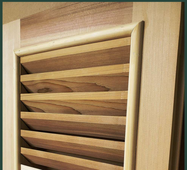
Rabbet Edge -or- Beaded Rabbet Edge
