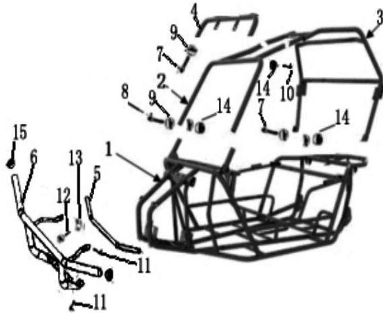
FIG 17. FRAME
