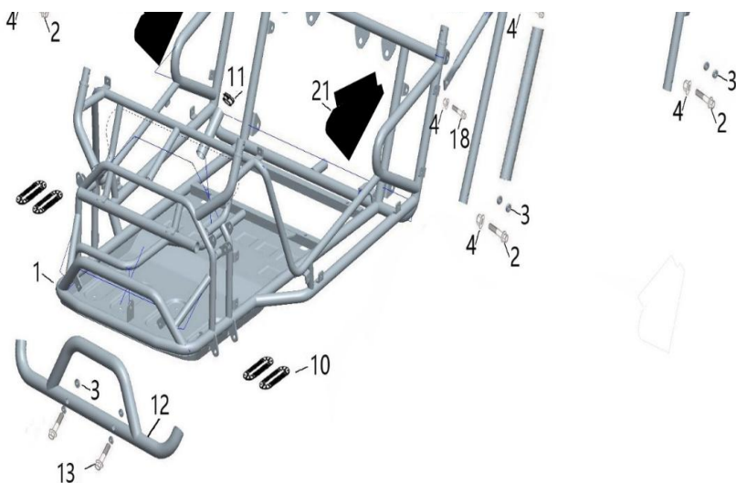
FIG:2 方向盘 STEERING WHEEL
