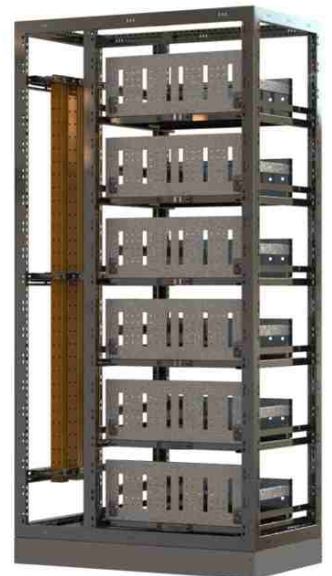
AÇIK TİP ŞALTER MODÜLÜ
