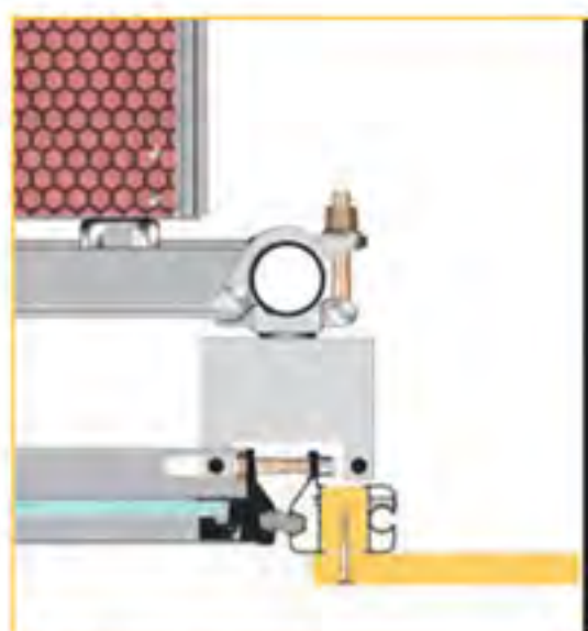
Sellado lateral a fachada
