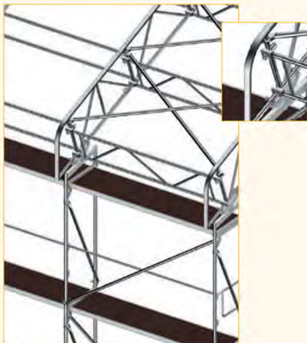
Detalle B: Rigidización en el plano de cubierta.
