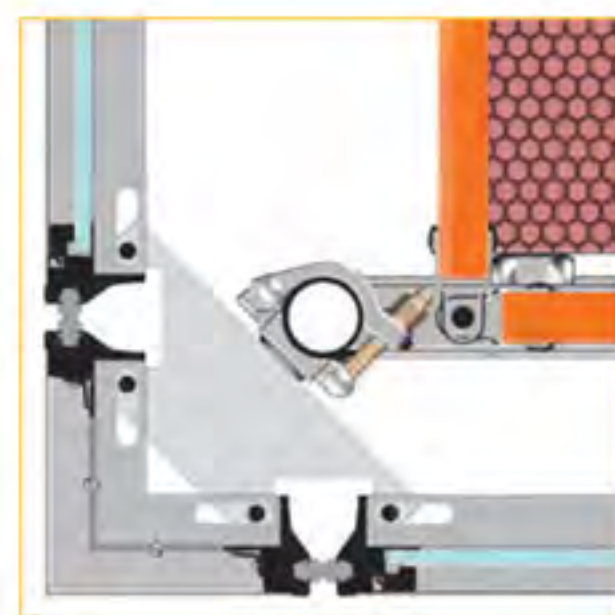
► Soporte Blitz para paneles de esquina
