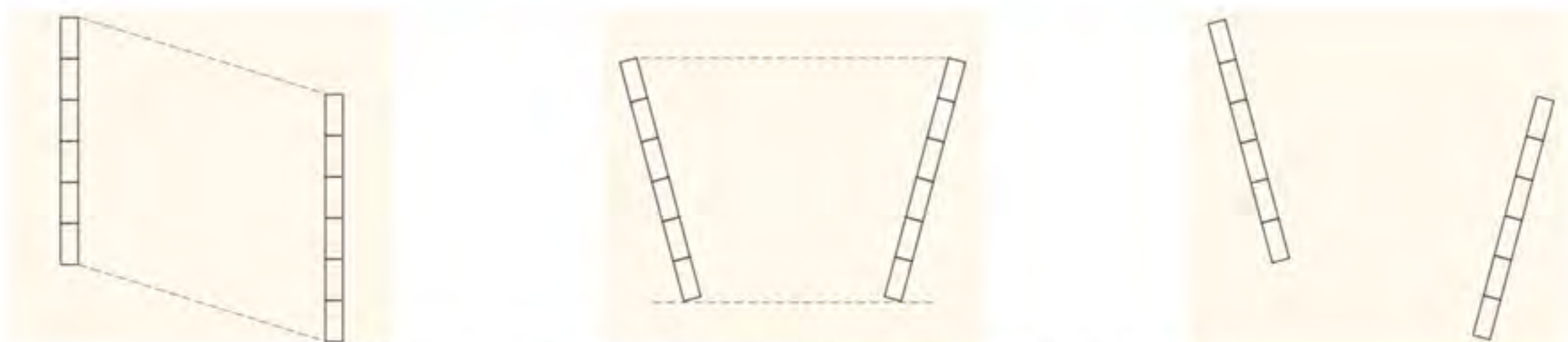
Posibles problemas en la alineación de los soportes que podrían provocar riesgos en la colocación de la cubierta
