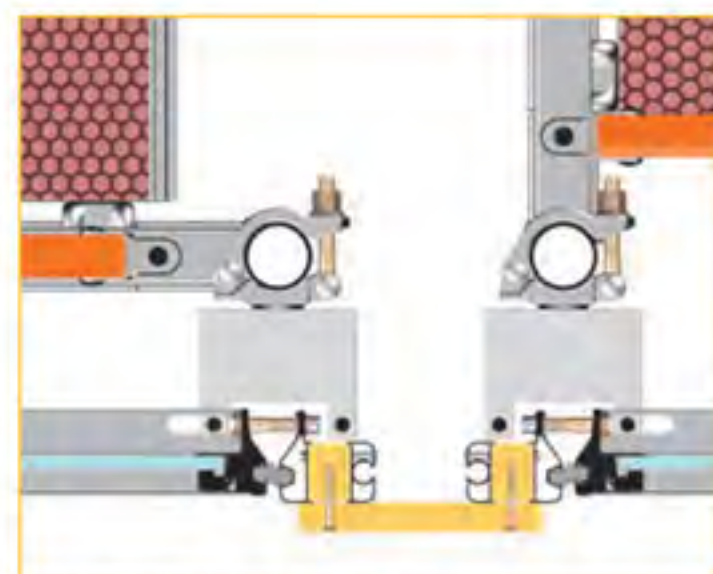
Sellado entre andamios independientes
