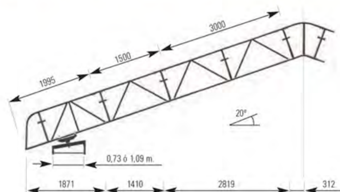
Sobre estructura de andamio (Allround o Blitz)
