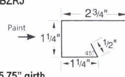
JAMB TRIM BZRJ
