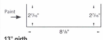
JAMB HEADER BZRJH
