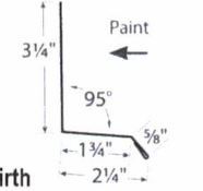
JAMB TRIM BZRJ
