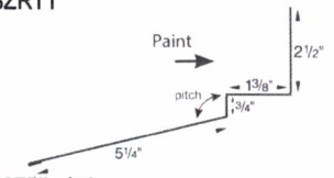
ZEE TRIM BZRZ
