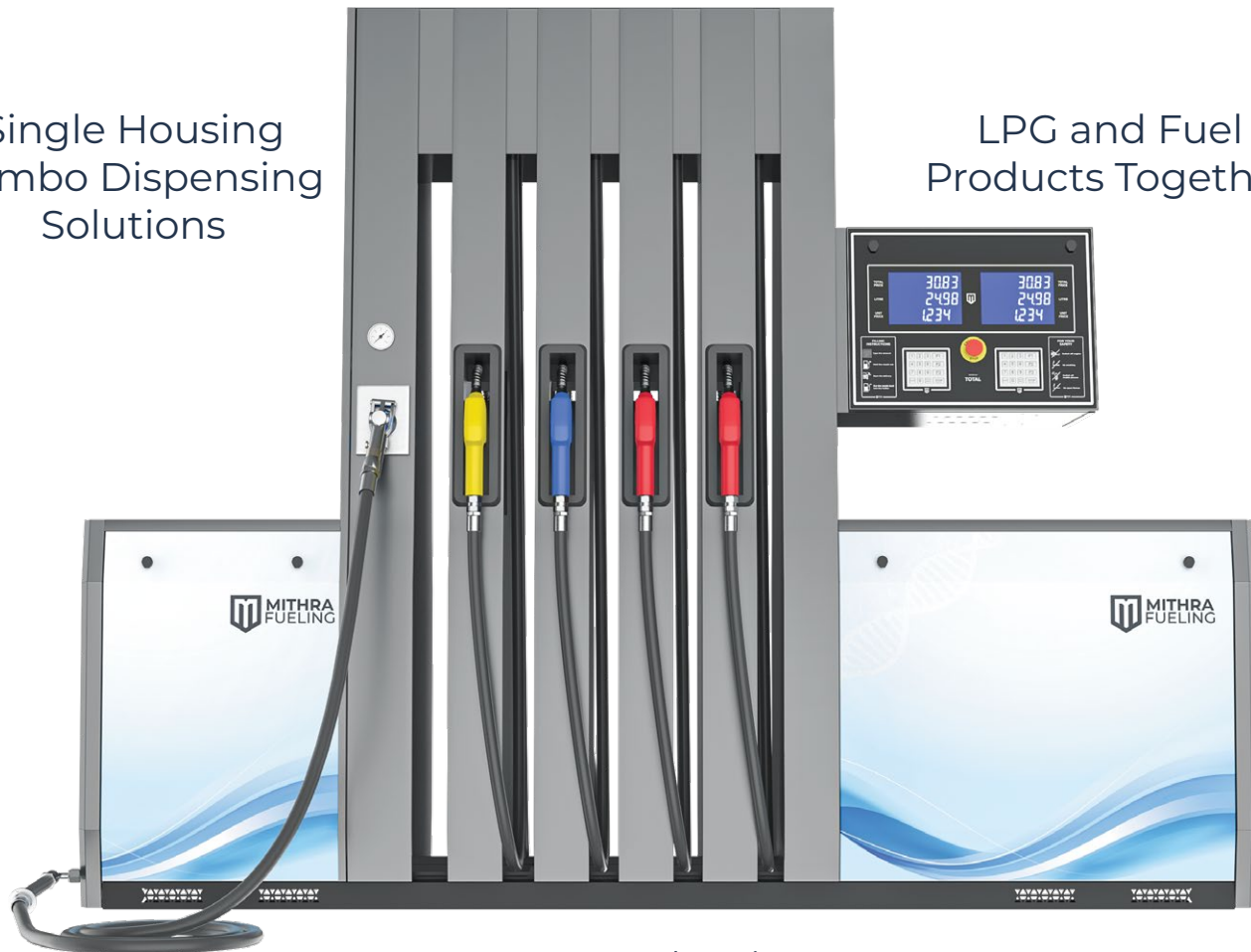
Inno 6000 H Combo Dispenser
