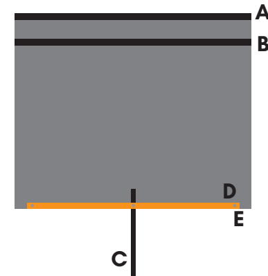
MUTCD R4-7A
