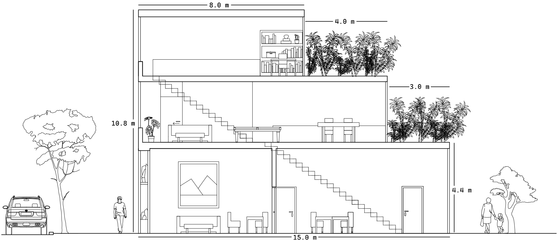
schnitt atelierhaus 1:100
