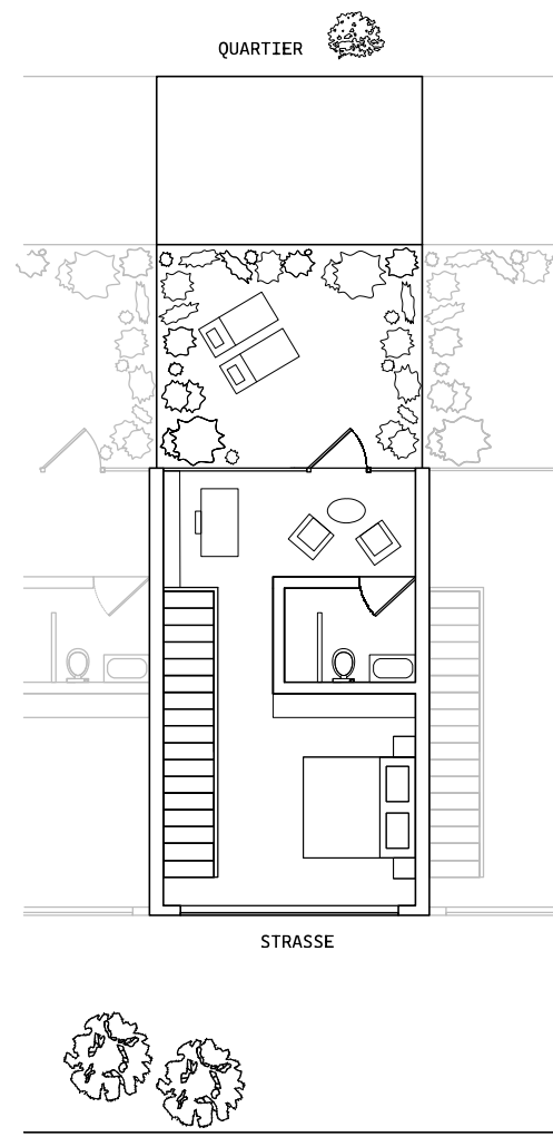
2. obergeschoss wohnen 1:100
