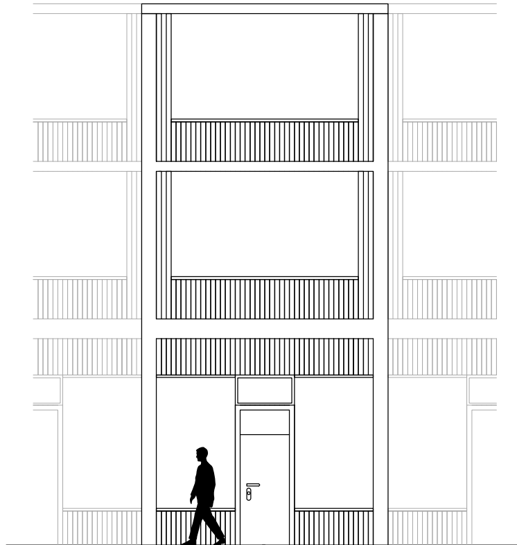
atelierhaus ansicht strasse 1:100
