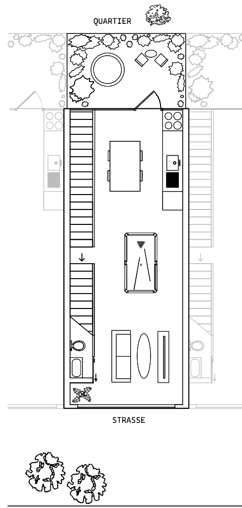
1. obergeschoss wohnen 1:100
