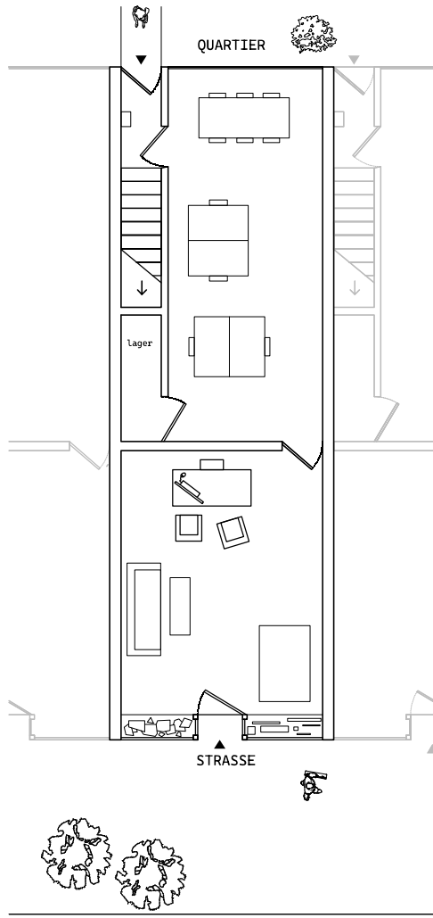
erdgeschoss arbeit 1:100
