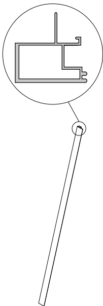
"Left Side Guide Profile"
