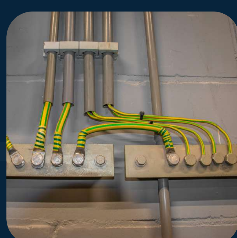
تأريض كهربائي لكامل المبنى
