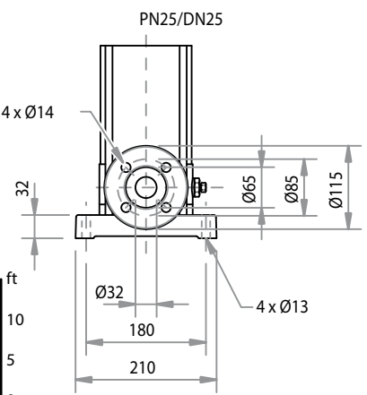
Dimensiones y Pesos
