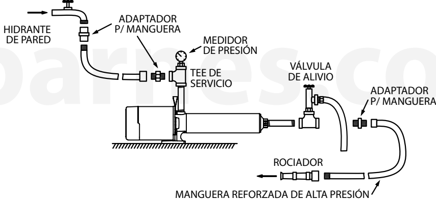
Figura 4: Bomba usada para aumentar la presión en un hidrante de pared (operación manual).
