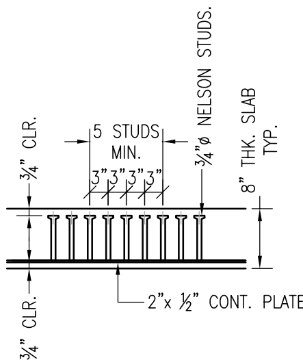
TYP. STUDRAIL LEG
