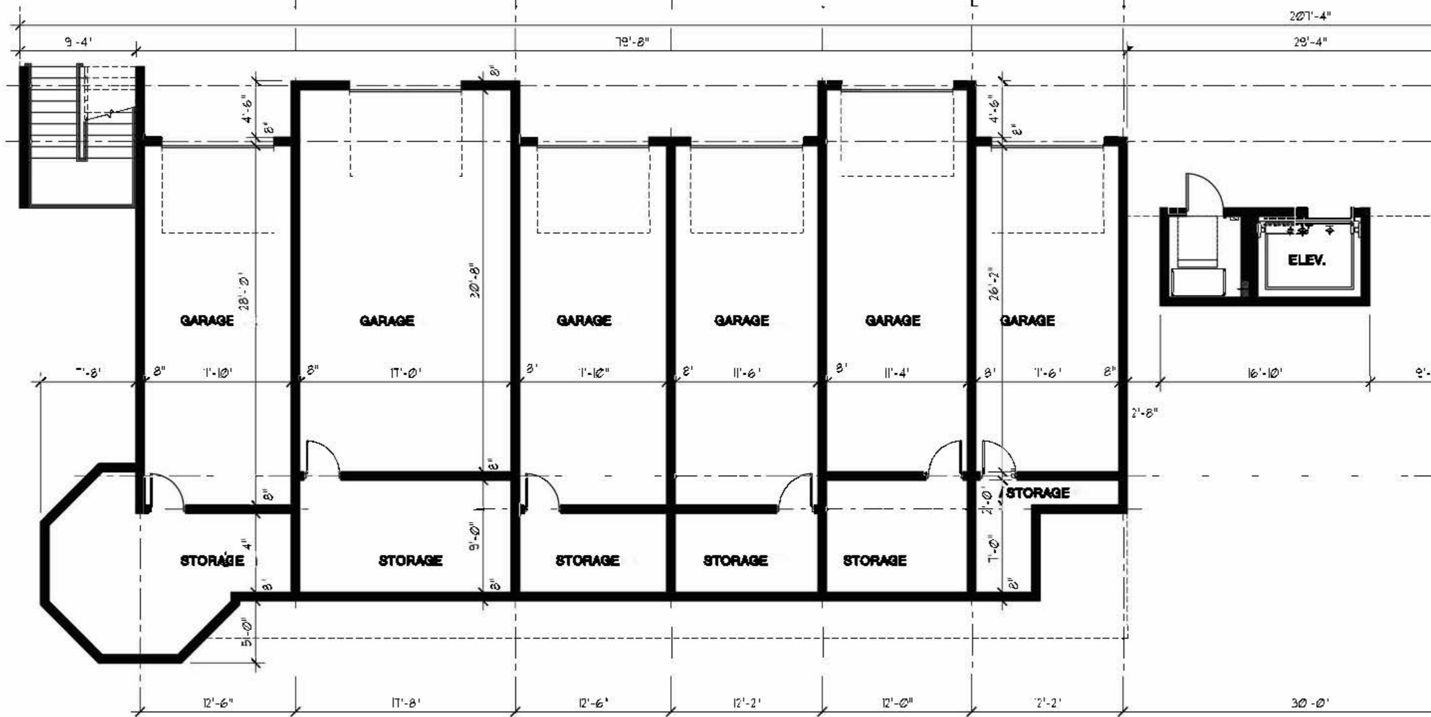
LOWER LEVEL PLAN SCALE: 1/8" = 1'-0"
