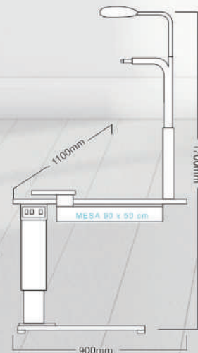
• Dimensión CP-180A
