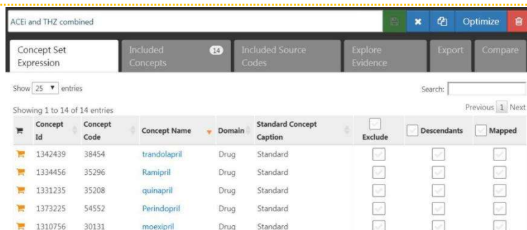
图 18.3: 一个包含目标概念和对比者暴露概念的概念集。
