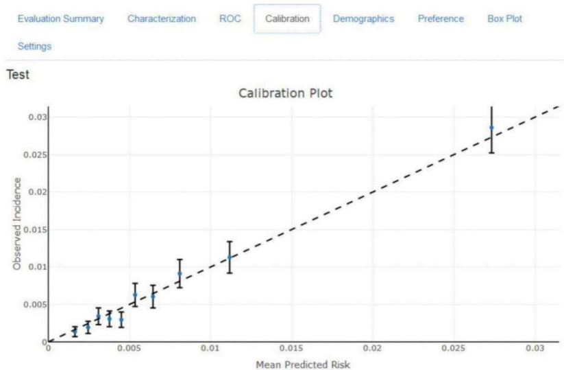
图 13.18: 模型校准
