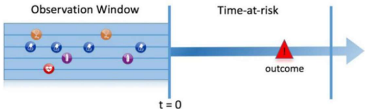
图 13.1 预测问题
