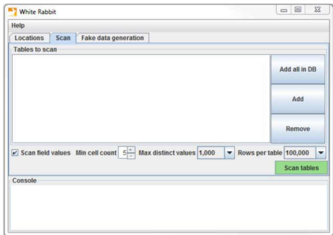
图 6.2: “White RabbitScan” 选项卡
