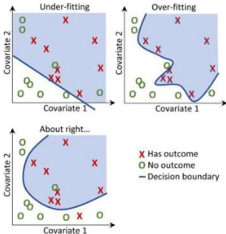
图 13.2: 决策边界
