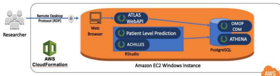
图 8.10: Amazon Web Services 中的 OHDSI-in-a-Box 架构
