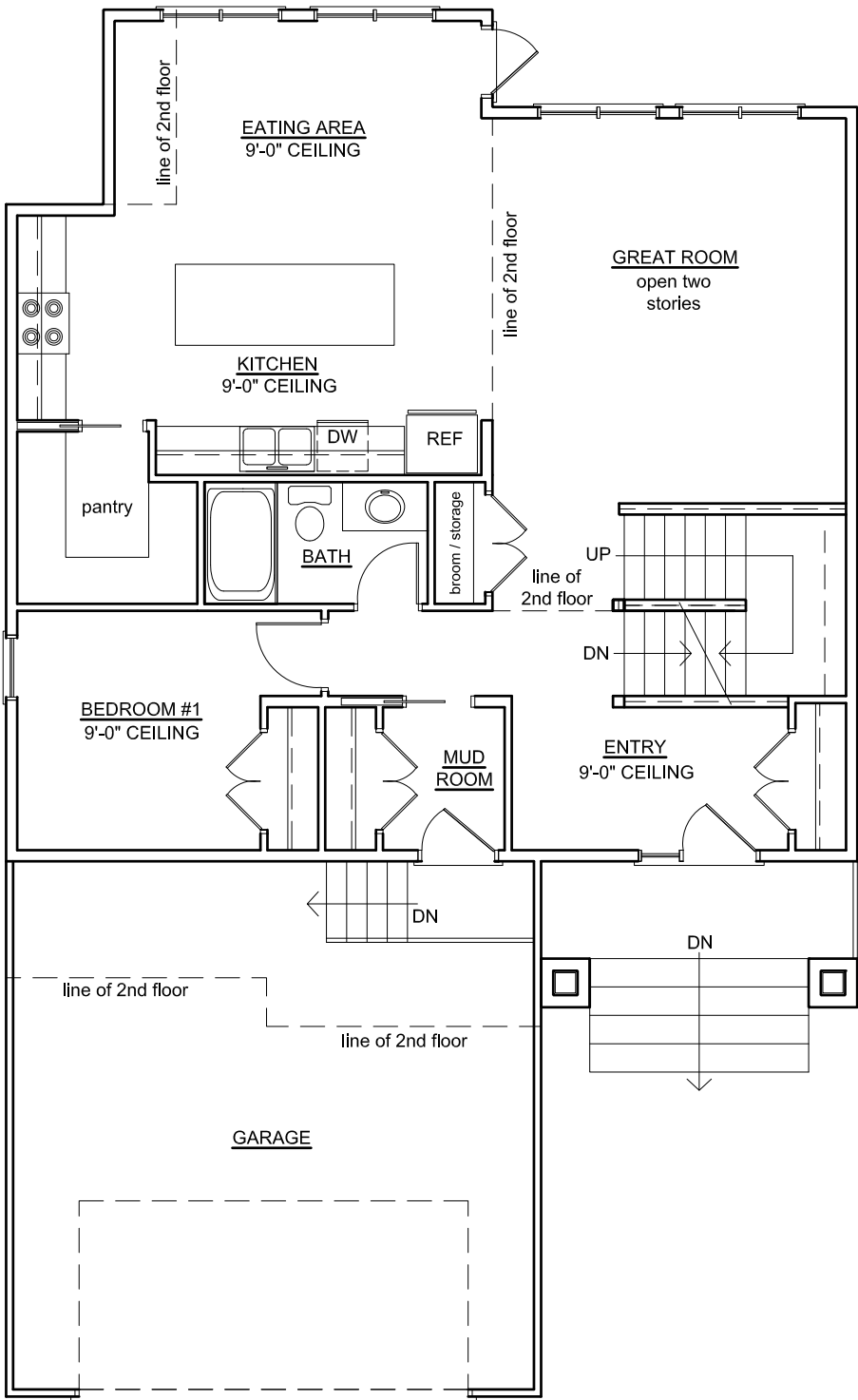
M A I N F L O O R P L A N
