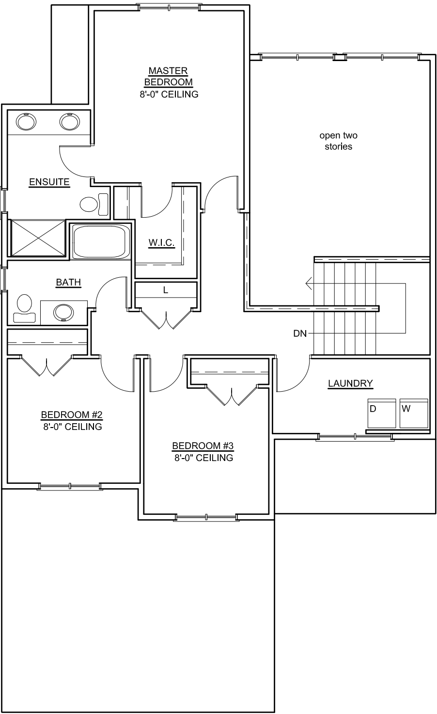
S E C O N D F L O O R P L A N
