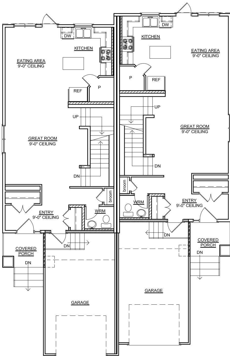
M A I N F L O O R P L A N S
