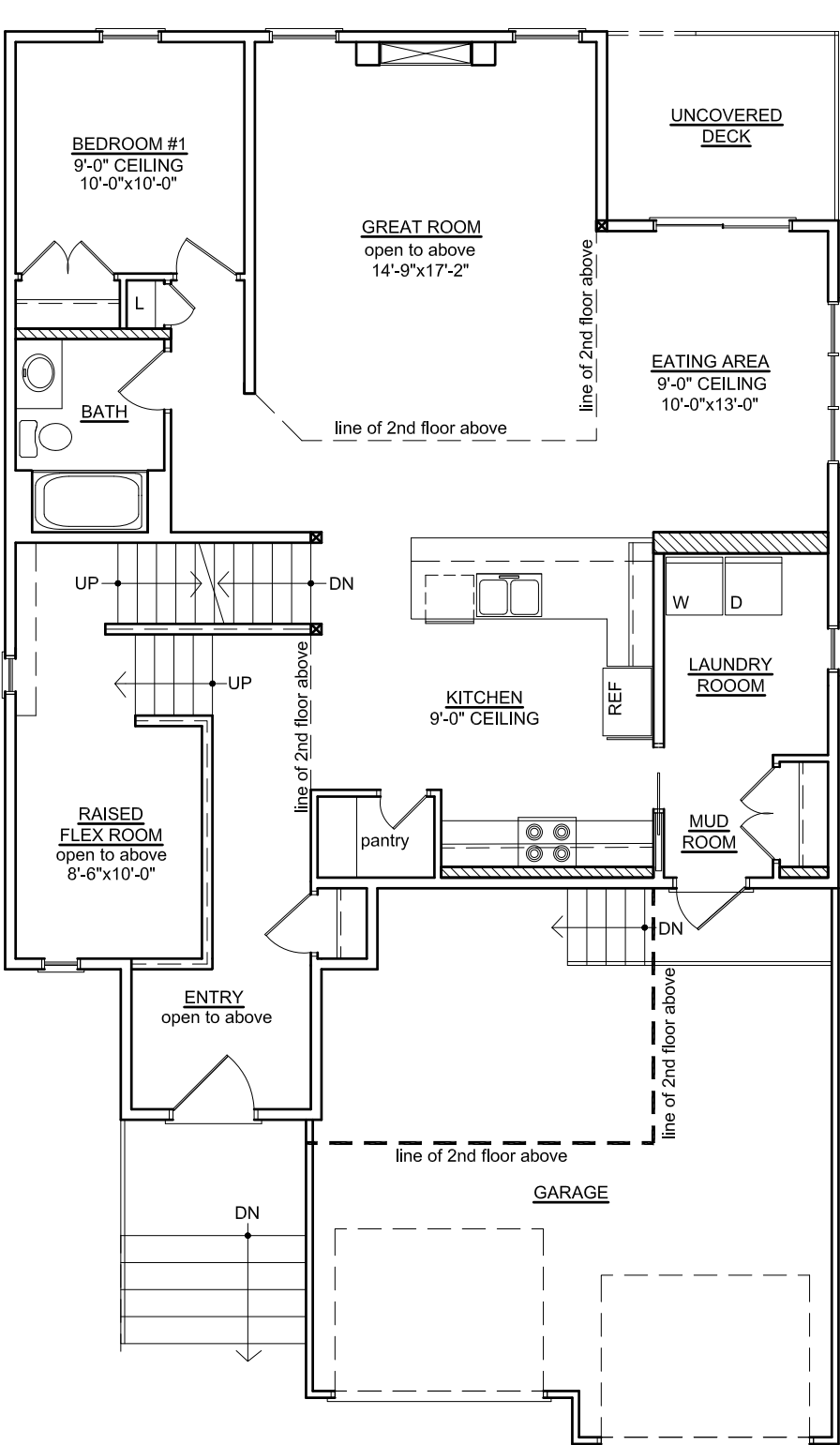
M A I N F L O O R P L A N
