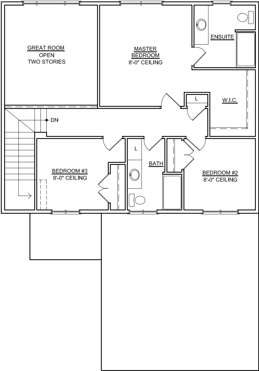
S E C O N D F L O O R P L A N
