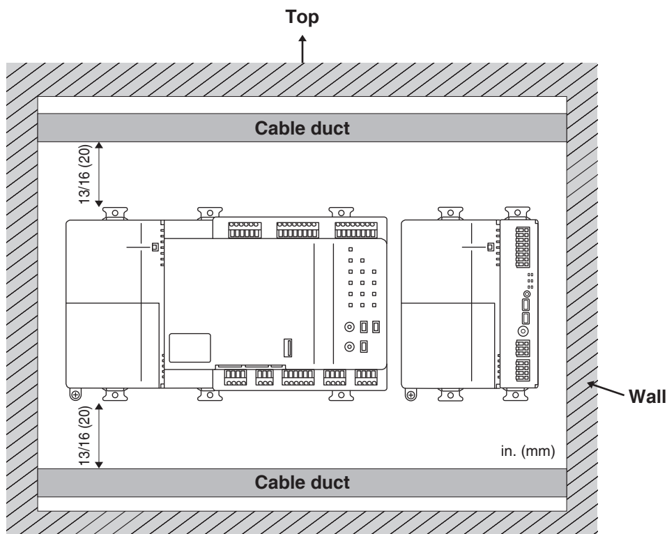
<Daikin HERO Pro Edge installation space>
