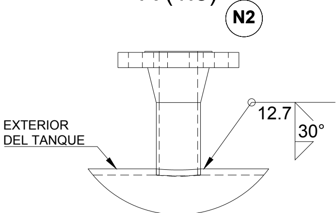
DETALLE BOQUILLA ENTRADA PURGA
