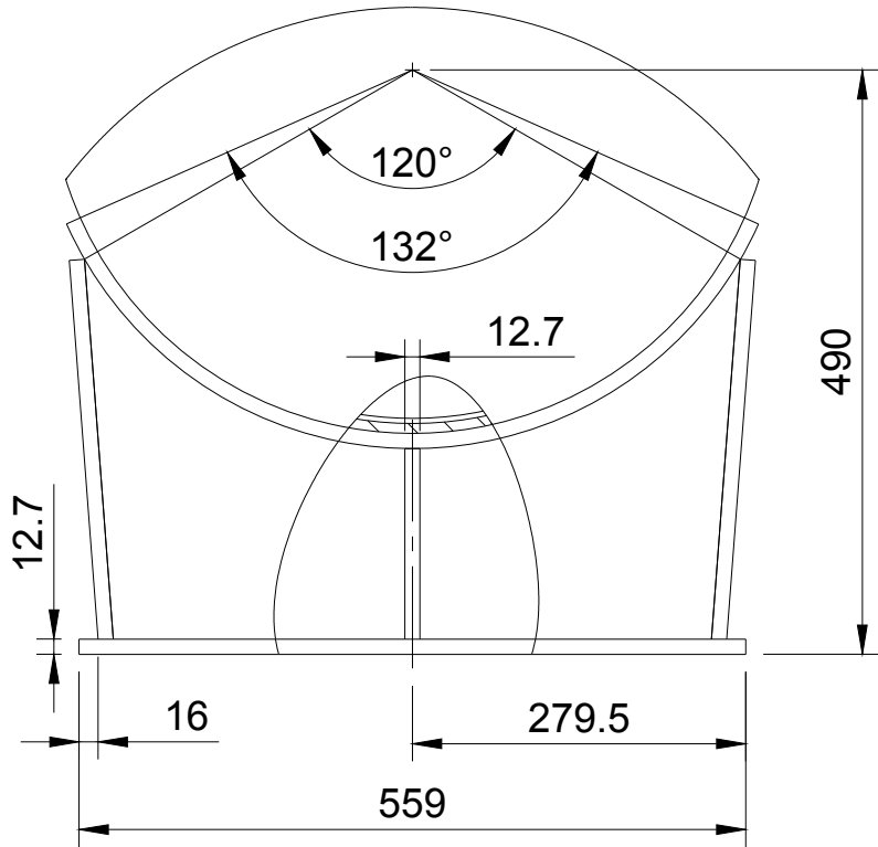
DETALLE SILLETA
