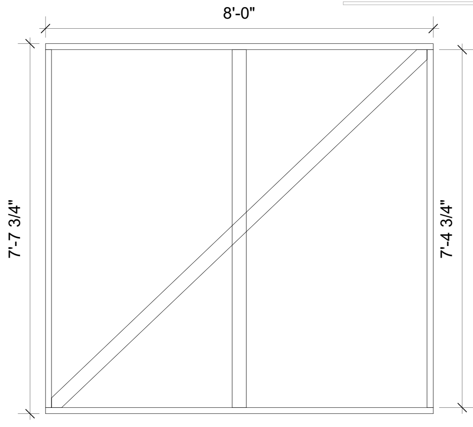
2 Frame 2 - Build 5 Scale: 1/2" = 1'-0"
