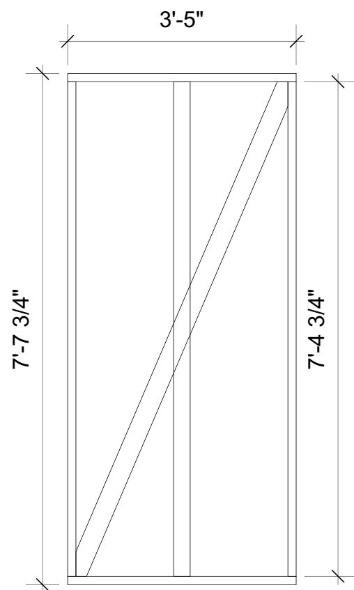
1 Frame 1 - Build 4 Scale: 1/2" = 1'-0"
