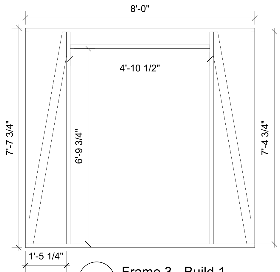
3 Frame 3 - Build 1 Scale: 1/2" = 1'-0"
