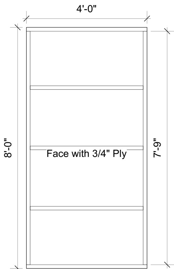
4 Flat 1 - Build 3 Scale: 1/2" = 1'-0"
