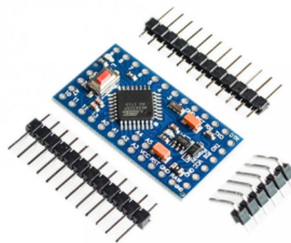
Arduino Pro Mini ATMEGA328P Compatible Board
