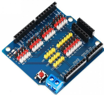
Arduino UNO R3 Sensor Shield V5.0
