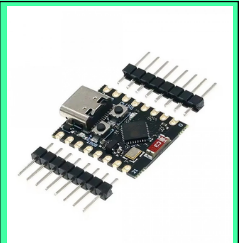
ESP32-C3 Super Mini Development Board
