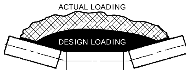
Fig 4: Actual versus design volumetric loading
