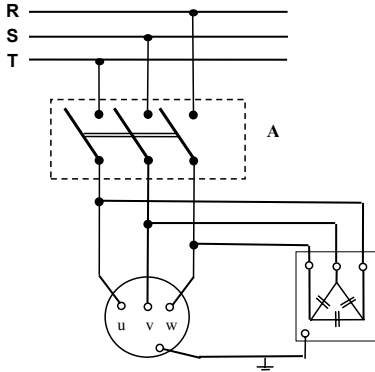
Doğrudan doğruya şebekeye bağlanan kısıadevre rotorlu bir asenkron motorun bireysel kompanzasyonu
