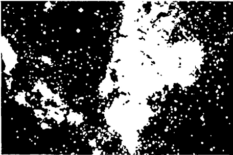
Resim 6 Gaz halindeki bir nebula
