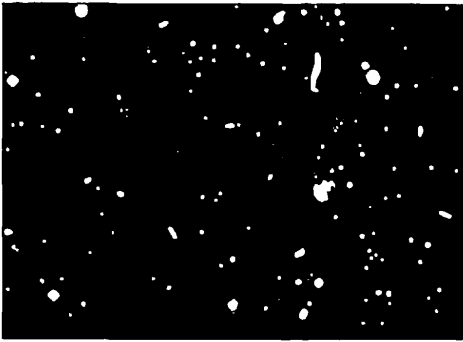
Resim 4 Bir galaksiler kümesi
